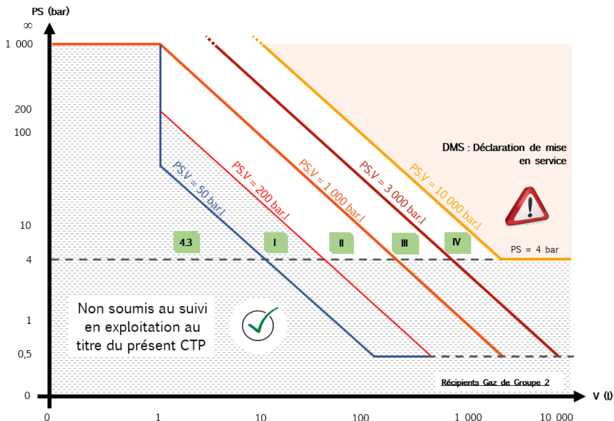
Extrait du Tableau 2 Annexe II de la Directive 2014/68/UE Réceptifs visés à l'article 4, paragraphe I point a), i) tiret deux
