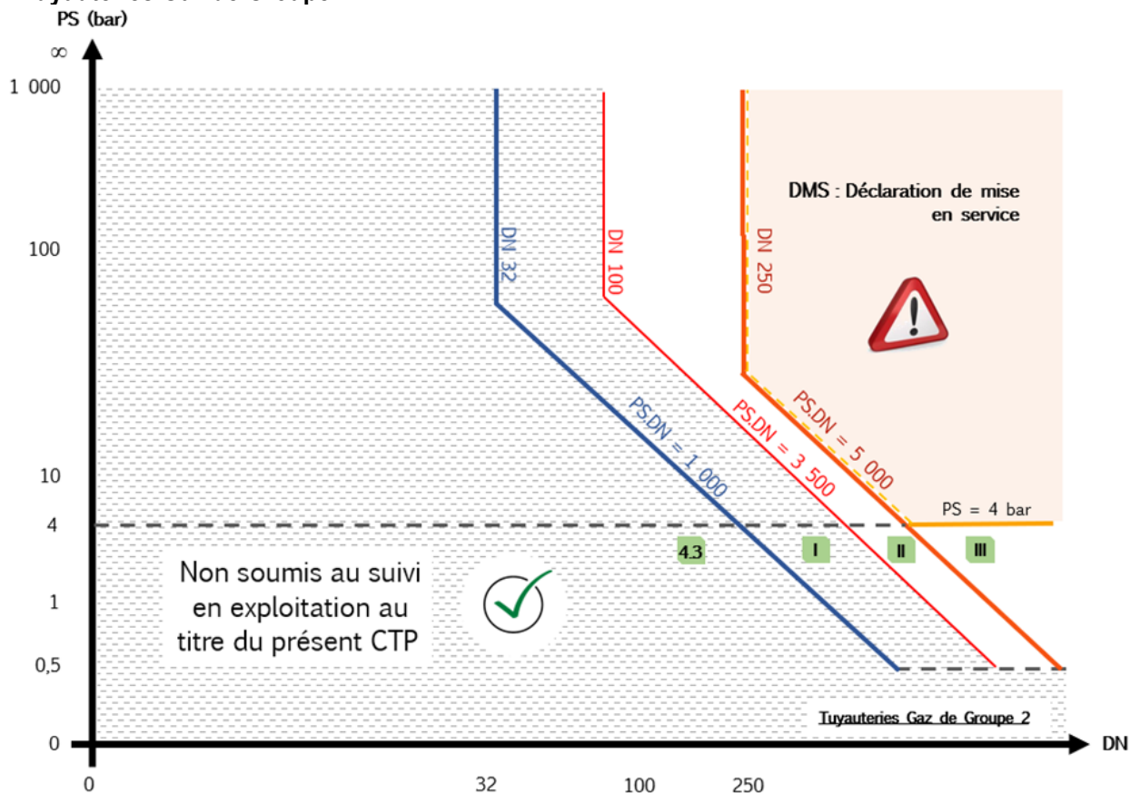
Extrait du Tableau 7 Annexe II de la Directive 2014/68/UE Tuyauteries visées à l'article 4, paragraphe I point c), i), tiret deux
