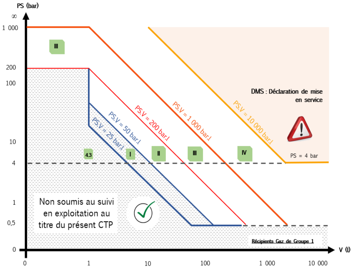
Extrait du Tableau 1 Annexe II de la Directive 2014/68/UE Réceptifs visés à l'article 4, paragraphe I point a), i) tiret un
