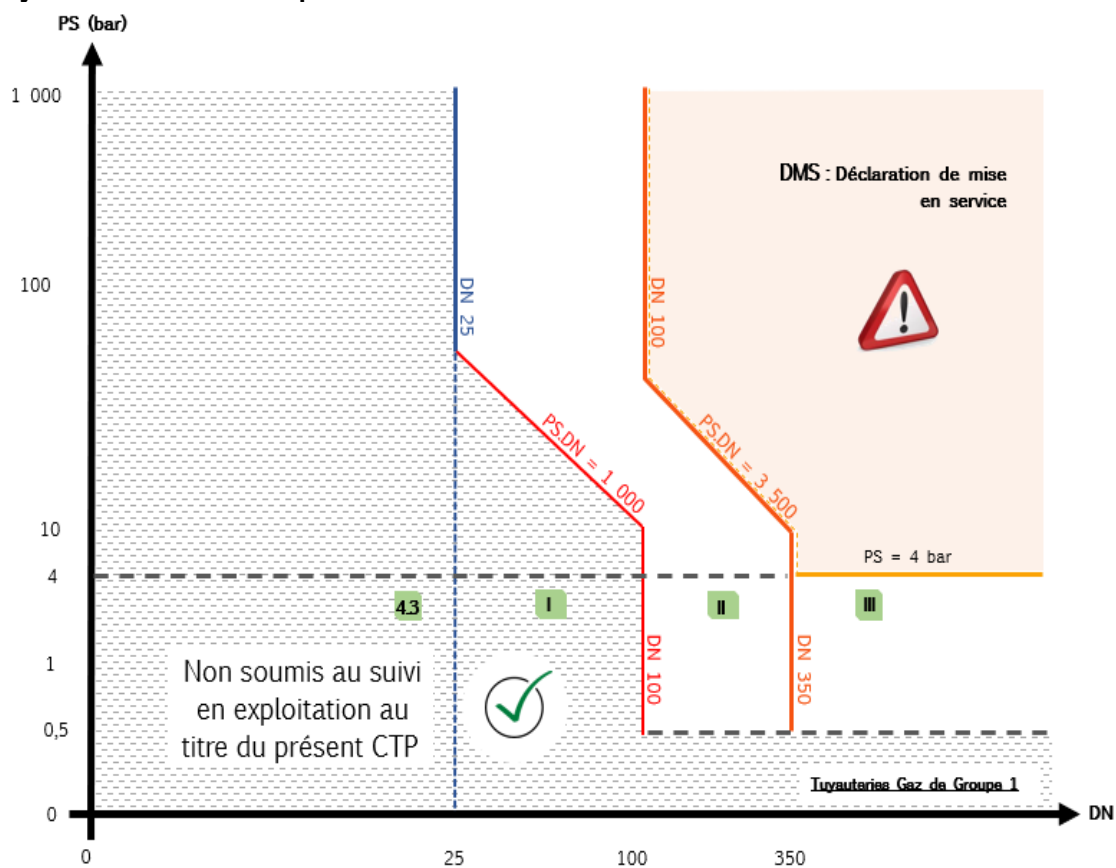
Extrait du Tableau 6 Annexe II de la Directive 2014/68/UE Tuyauteries visées à l'article 4, paragraphe I point c), i) tiret un
